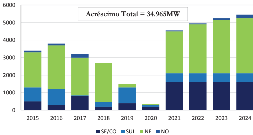
Acréscimo de Capacidade Instalada de Eólica, PCH, Biomassa e Solar
